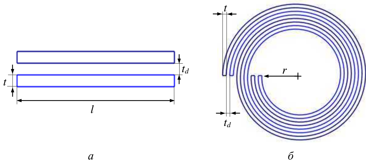
Рис. 23. Поперечные сечения прямоугольной (а) спиральной (б) шин питания
