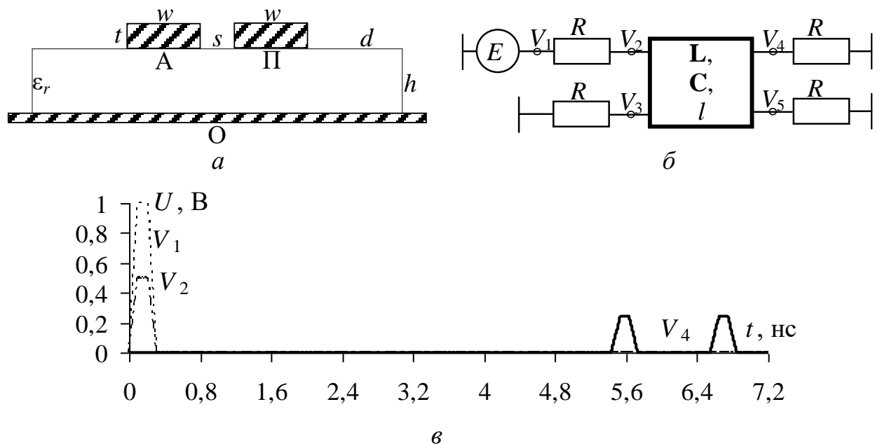
Рис. 1. Поперечное сечение (а), эквивалентная схема (б) и формы ЭДС ( V_1 ), напряжения на входе ( V_2 ) и выходе ( V_4 ) (в) МФ на основе связанной МПЛ
