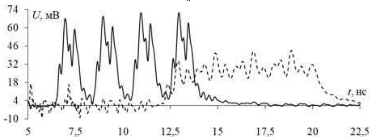
Рис. 17. Формы напряжений на выходе зеркально-симметричных МФ (—) и МЛ (---) при воздействии пачки СКИ с периодами повторения 0,5 (а), 1 (б) и 2 нс (в)
