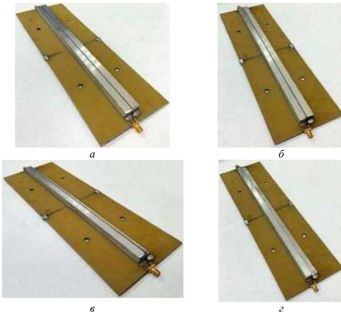
Рис. 10. Внешний вид МФ с пассивным проводником: сплошным (а), полым (б), уголковым (в), тонким (г)
