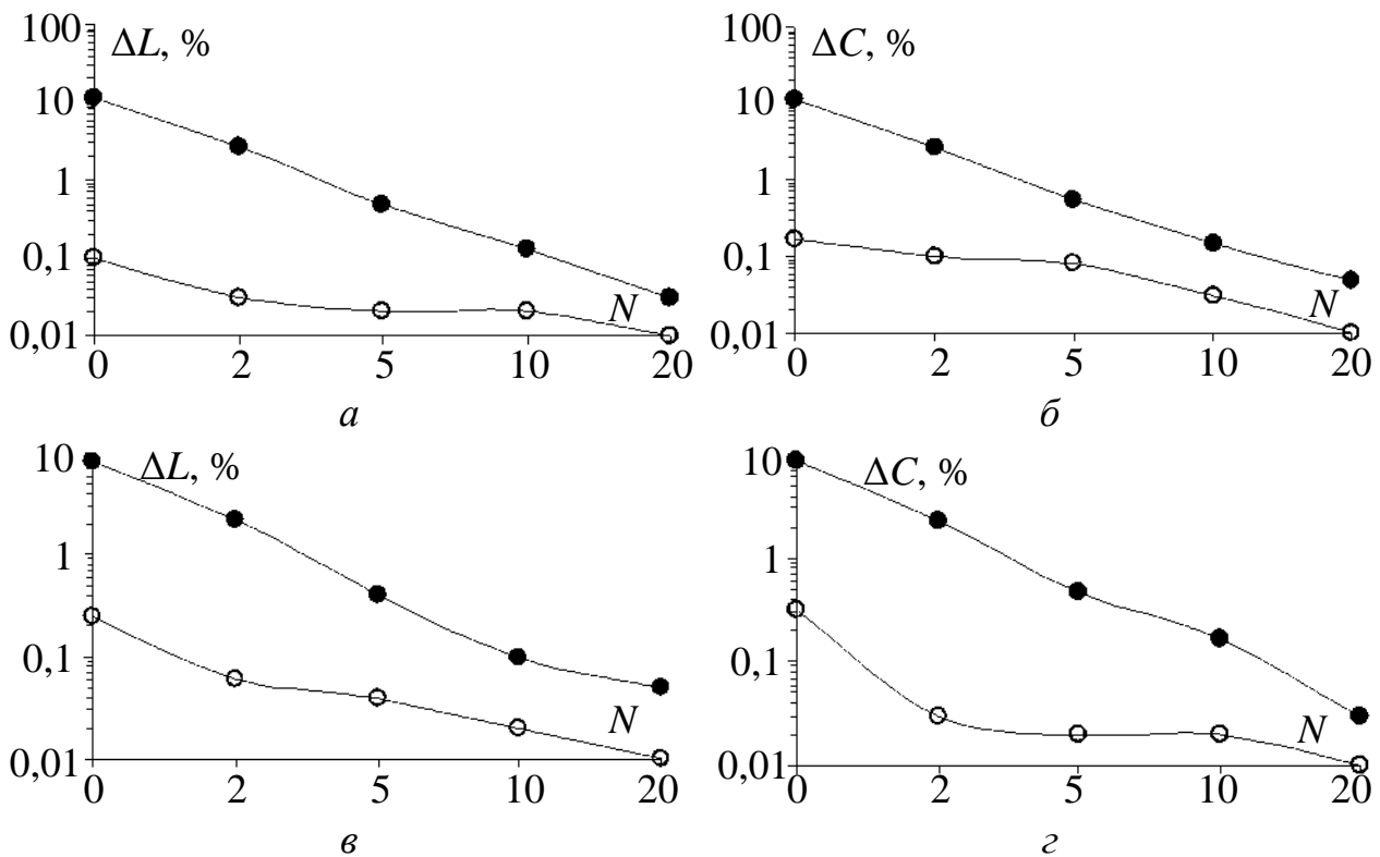
Рис. 22. Относительная погрешность вычисленных значений погонных L ( a, в ) и C ( б, г ) без сдвига пластин толщиной t \rightarrow 0 ( a, б ) и t=0,1 мм ( в, г ) при r/w=0,01 (●) и r/w=100 (○)
